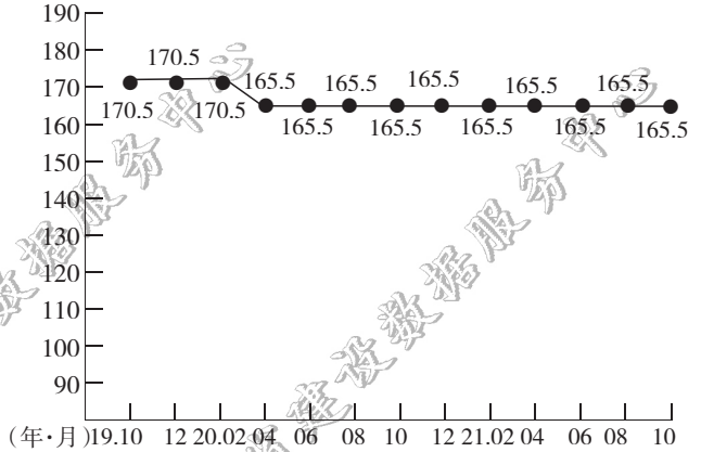
(元/m³) 碎石
